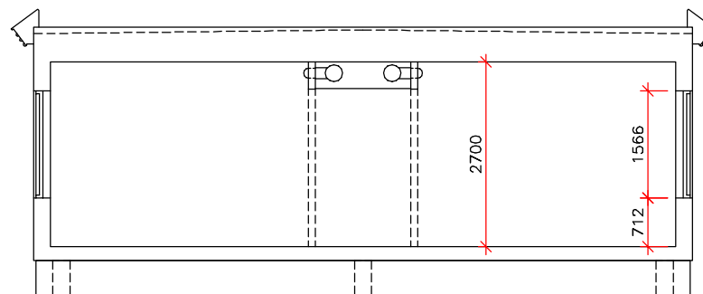
SEKTION
